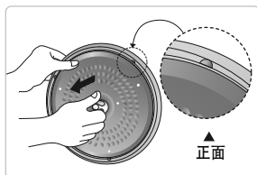
分离式内锅盖手柄从背面插入并在分离式内锅盖正面像箭头方向打动即可安装。
